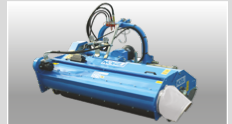
Coclea singola per la pacciamatura da un solo lato. Single spiral for mulched stubble delivery on one side.
